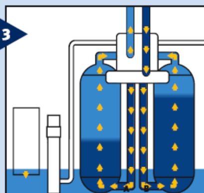
Después de la regeneración, las dos botellas descalcifican.
