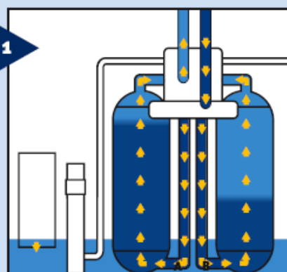
En servicio, las dos botellas dan agua descalcificada.
